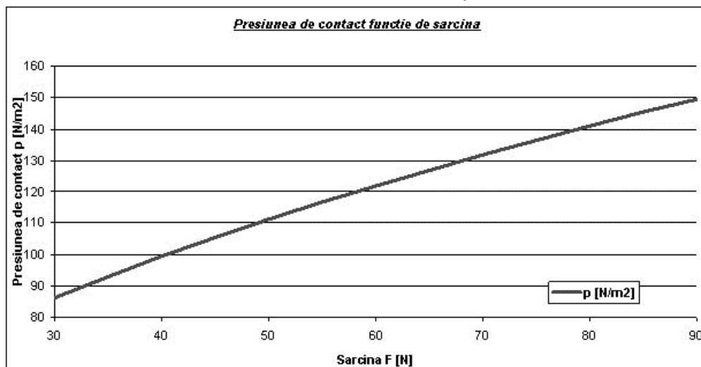
Graficul nr. 5: Presiunea de contact functie p functie de sarcina
