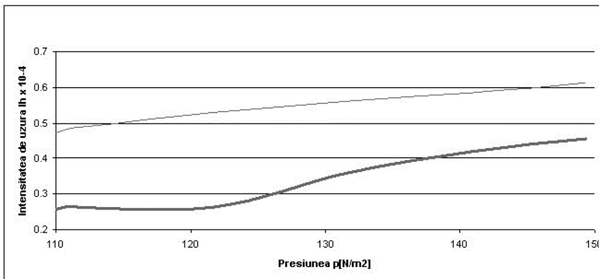
Graficul nr. 4: Intensitatea de uzura I_h \times 10^{-4} în funcție de presiunea de contact p , la n=400\text{rot/min}
