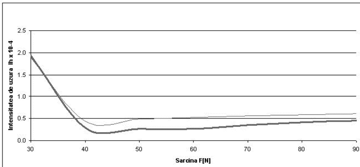
Graficul nr. 2: Intensitatea de uzura I_h \times 10^{-4} în funcție de sarcina N , la n=400\text{rot/min}
