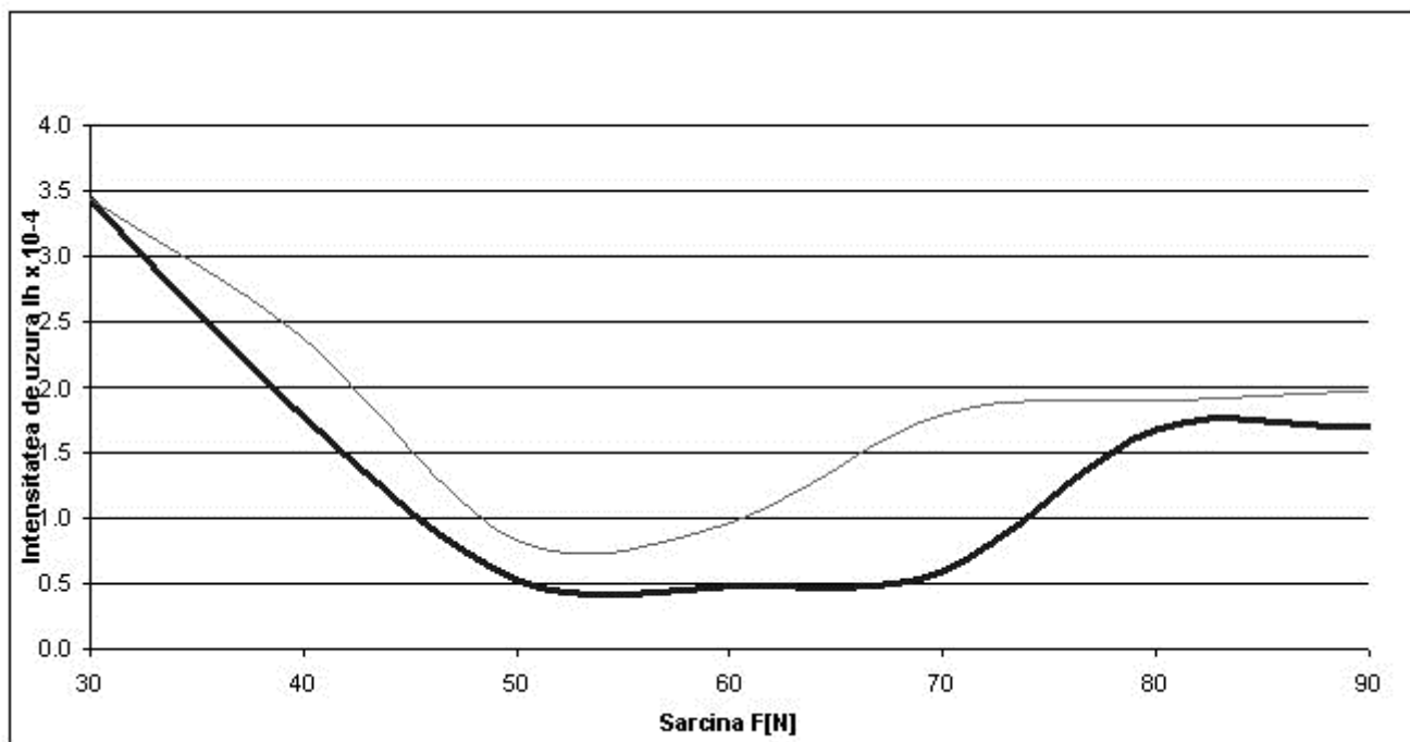
Graficul nr. 1: Intensitatea de uzura I_h \times 10^{-4} in functie de sarcina N, la n=200rot/min
