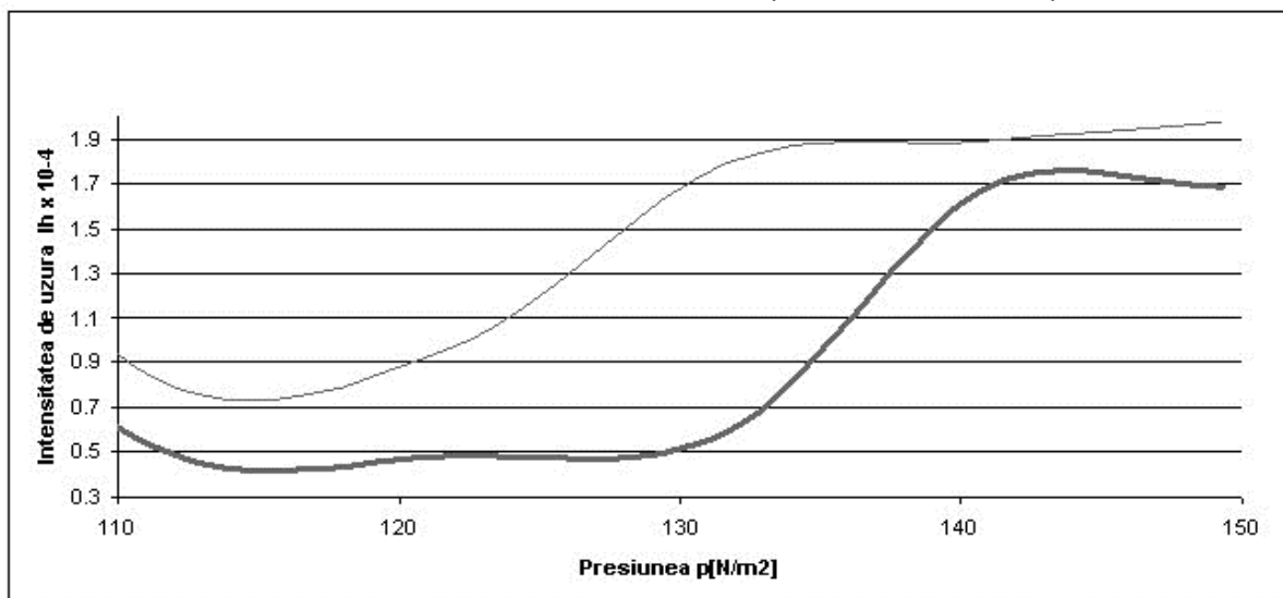
Graficul nr. 3: Intensitatea de uzura I_h \times 10^{-4} în funcție de presiunea de contact p , la n=200\text{rot/min}
